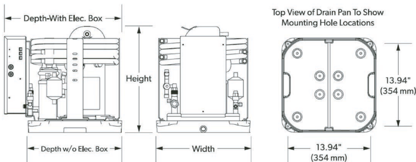
Dimensions DEUX24-72
