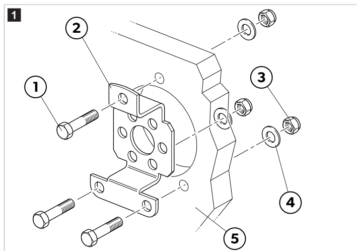
Support à 90°
