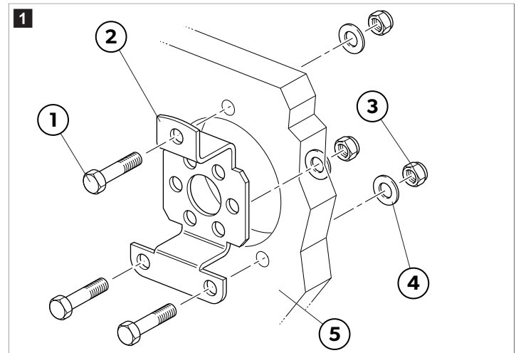
Staffa a 90°
