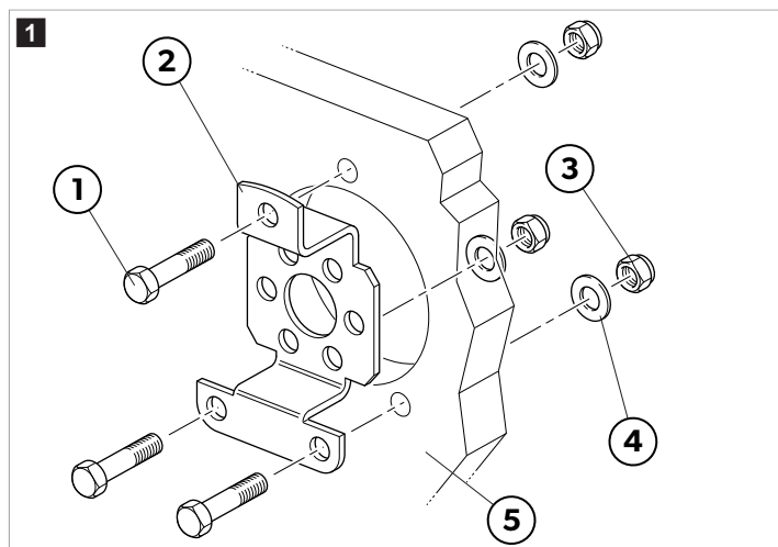
90° držák
