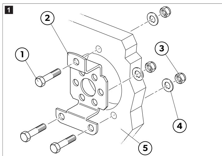
90° beslag
