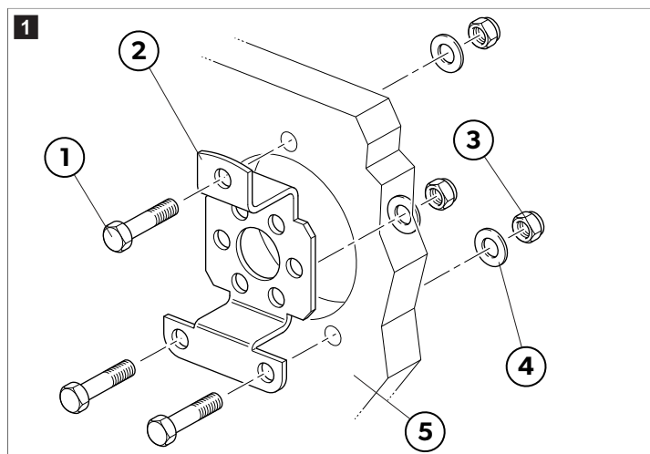
90° laikiklis
