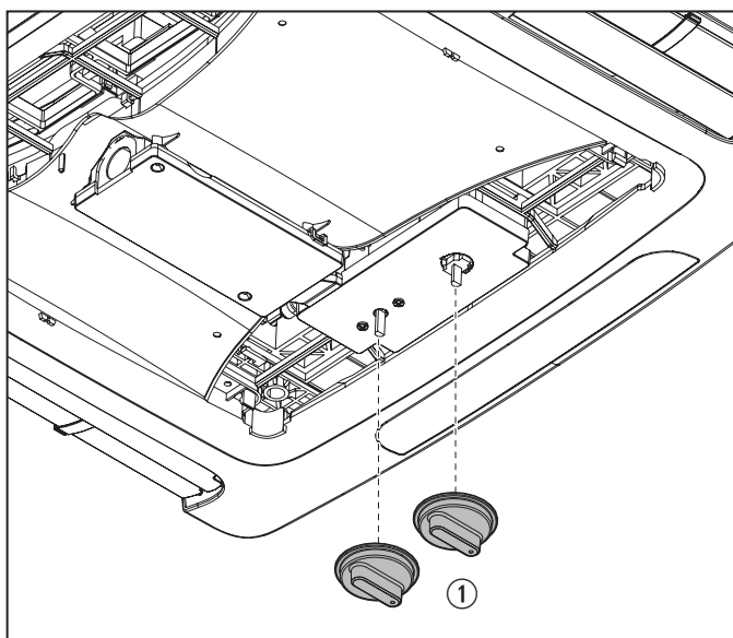
28 Fijación de las perillas de control
