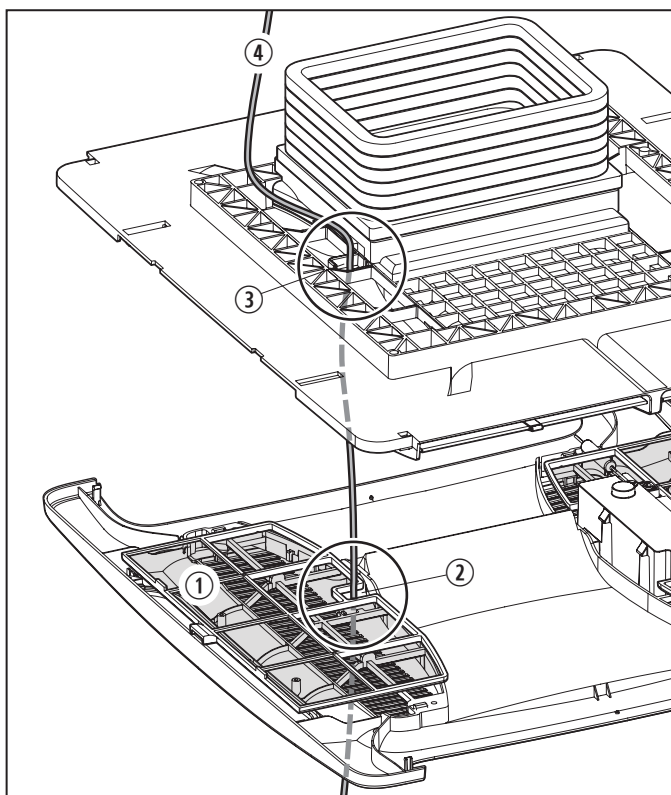
23 Pasar el cable por la muesca del filtro
