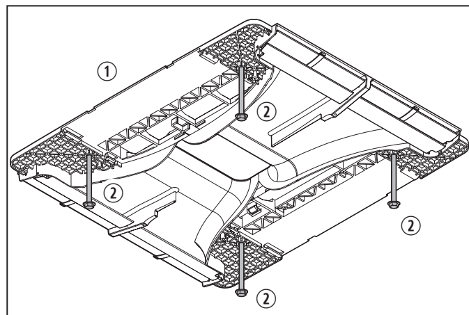
25 Ubicación de los pernos de montaje - Todos los modelos
