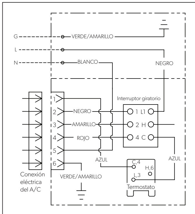
14 Diagrama de cableado de la ADB - Todos los modelos
