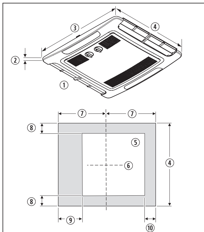
9 Medidas de las dimensiones
