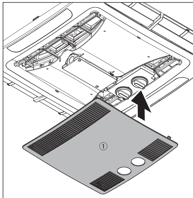
29 Fijación de la cubierta central
