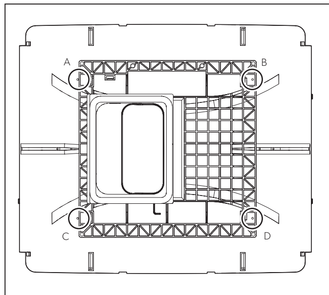
24 Patrón de montaje de pernos - Todos los modelos
