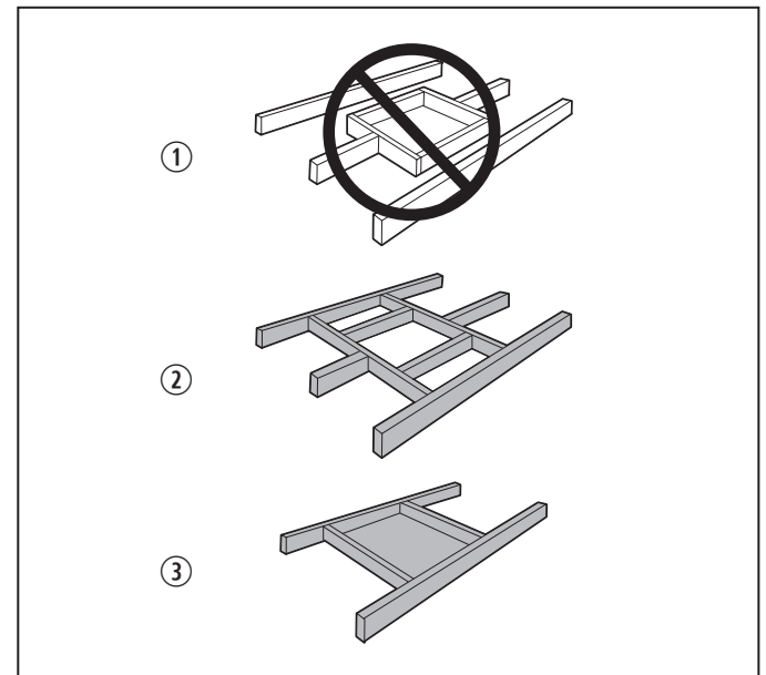
15 Estructura para una nueva abertura en el techo
