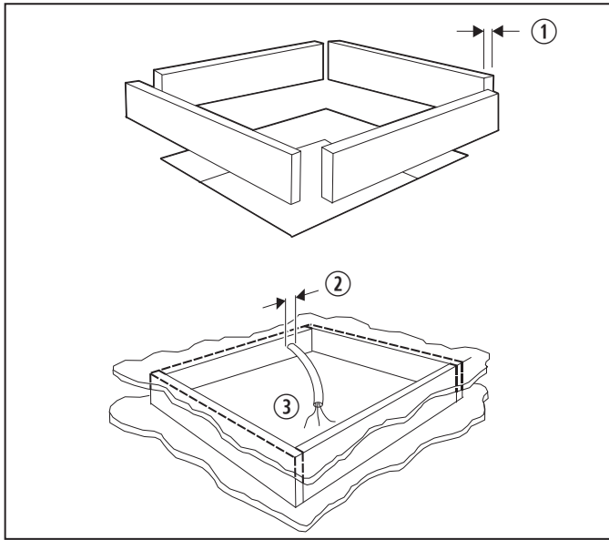
16 Marco estructural para una nueva abertura en el techo
