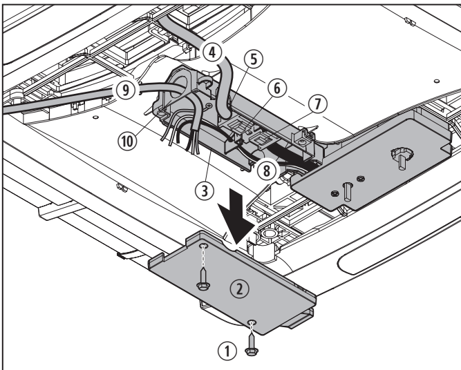
26 Finalización del cableado
