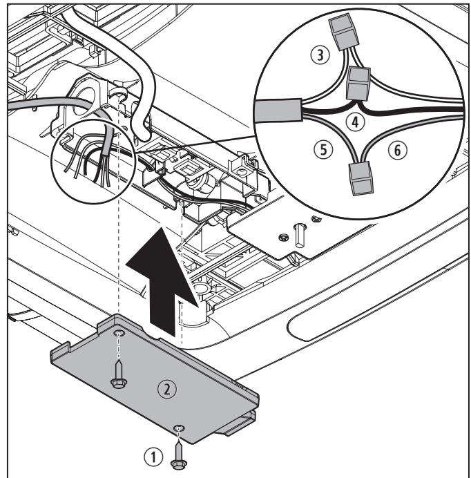
27 Caja de conexiones
